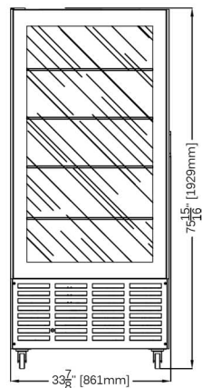
VC8314 H76
