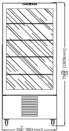
VC8314 H76
