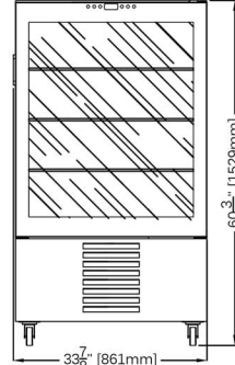
VII8314 H60
