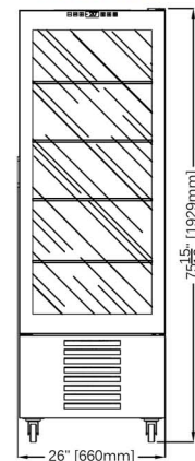
VN6314 H76
