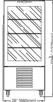
VII6314 H60
