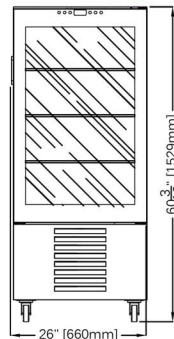
VN6314 H60
