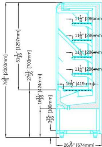
CU TYPE
